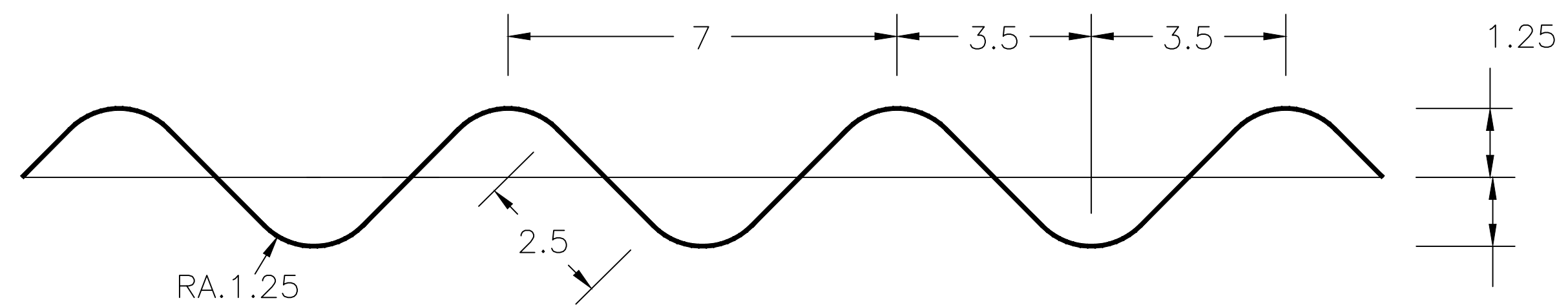
DETALLE DEL CORRUGADO DE LA LOSA
