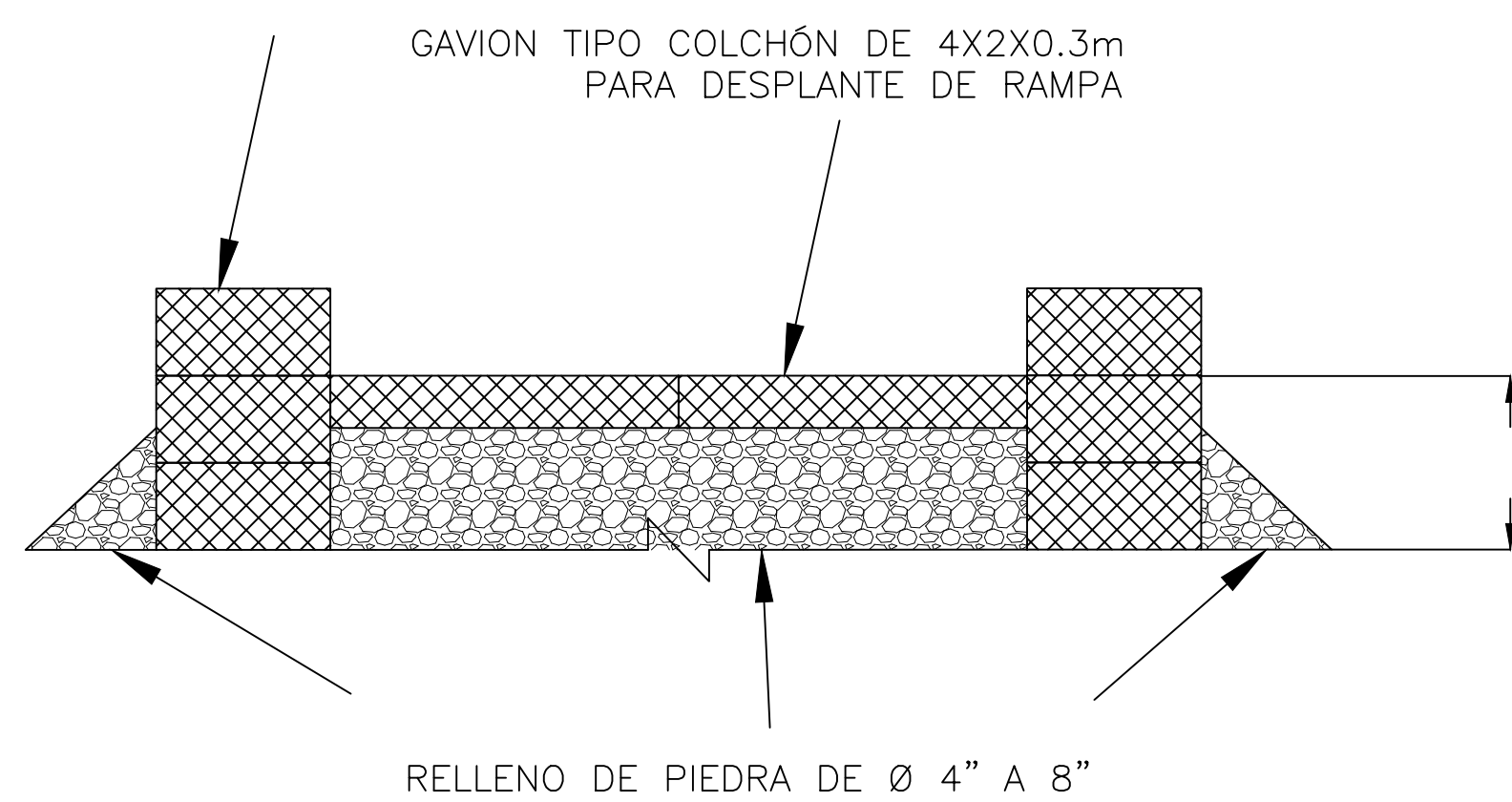
CORTE B-B'
