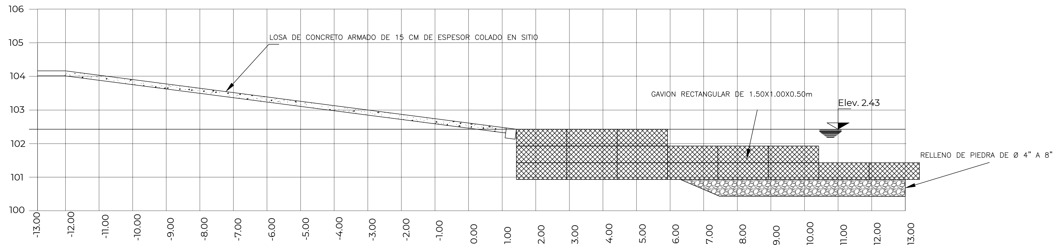
CORTE A-A'
