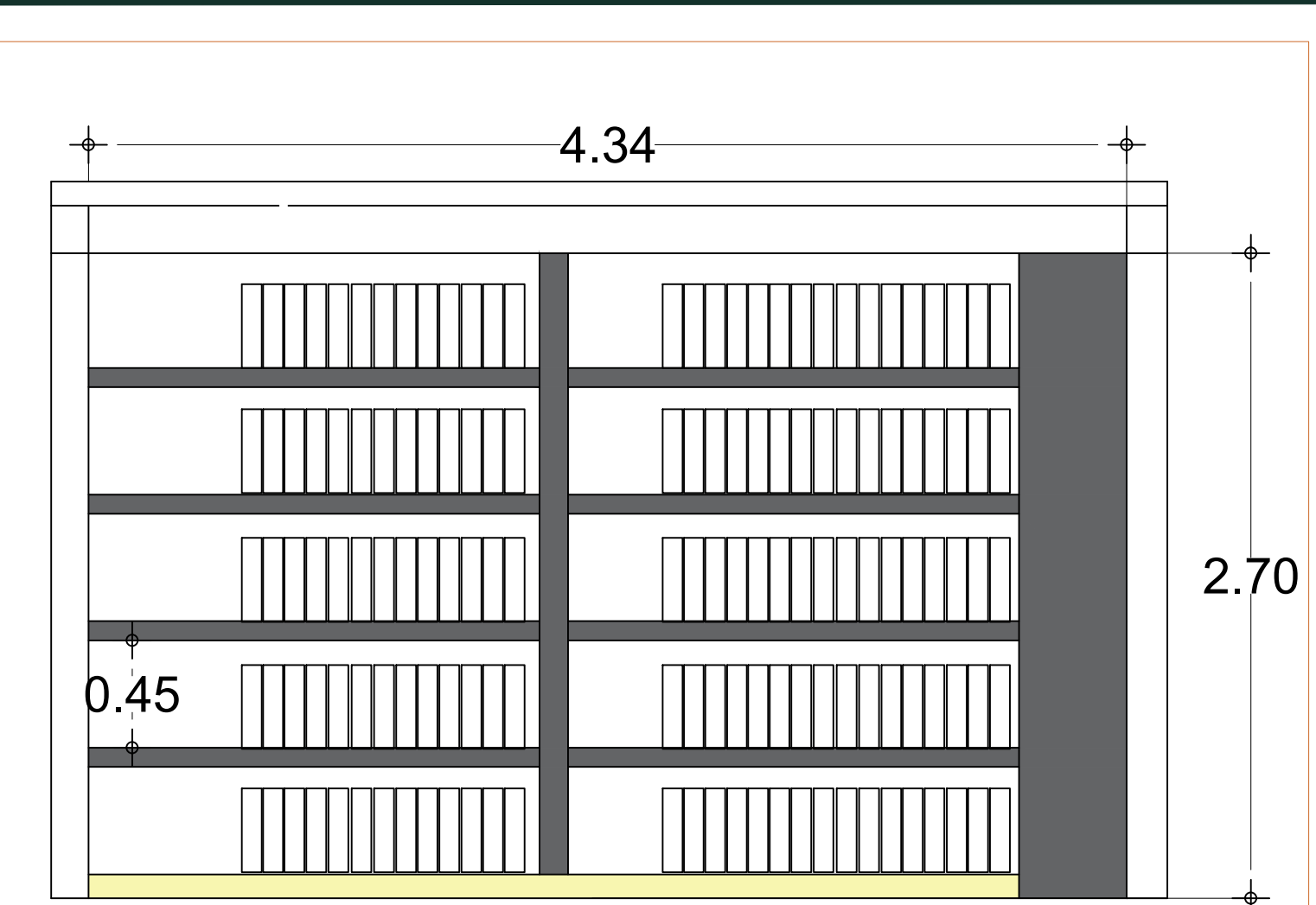
MUEBLE ARCHIVERO COLOCADO EN AREA MATRICULAS EN FORMA DE L 2.70 X 3.89 X .45
