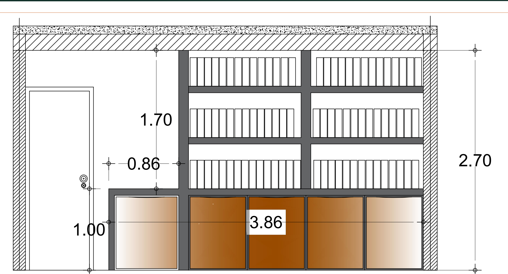
MUEBLE DE AREA OFICINA 2.70 X 3.86 X .45 ACABADO FORRO CON FORMAICA COLOR CHERRY HEARTWOOD.
