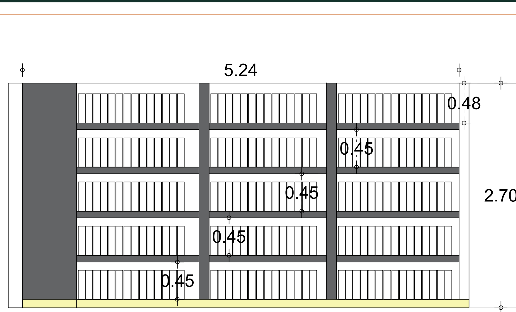
MUEBLE ARCHIVERO COLOCADO EN AREA REMAFE EN FORMA DE L 2.70 X 5.24 X .45 PINTADO COLOR GRIS
