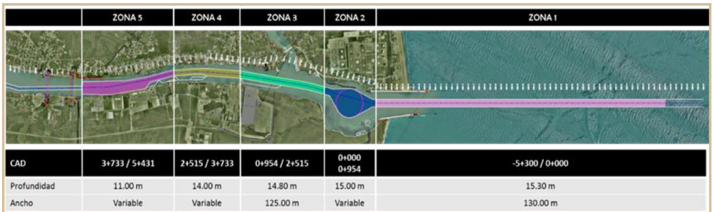
Imagen 1. Vista en planta del Canal de Navegación donde se realizarán los trabajos.
