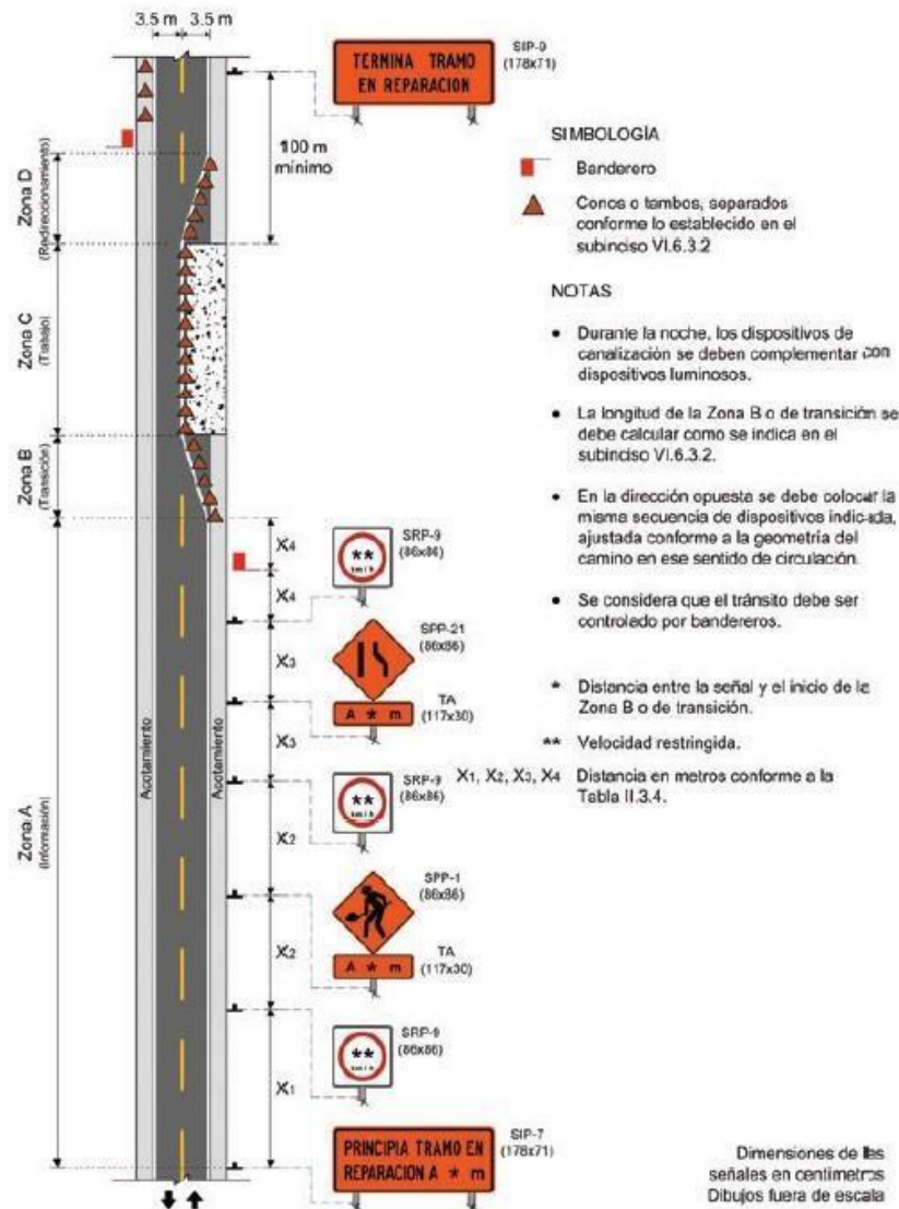
Figura VI-17. Ejemplo de señalización del cierre de un carril en carreteras con arroyo vial de un carril por sentido de circulación
